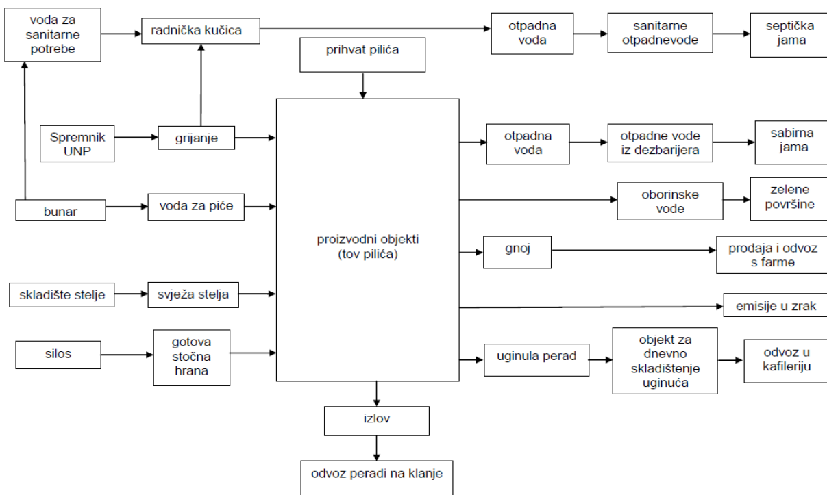
Prilog 3: Pojednostavljena shema procesa na Farmi 1
