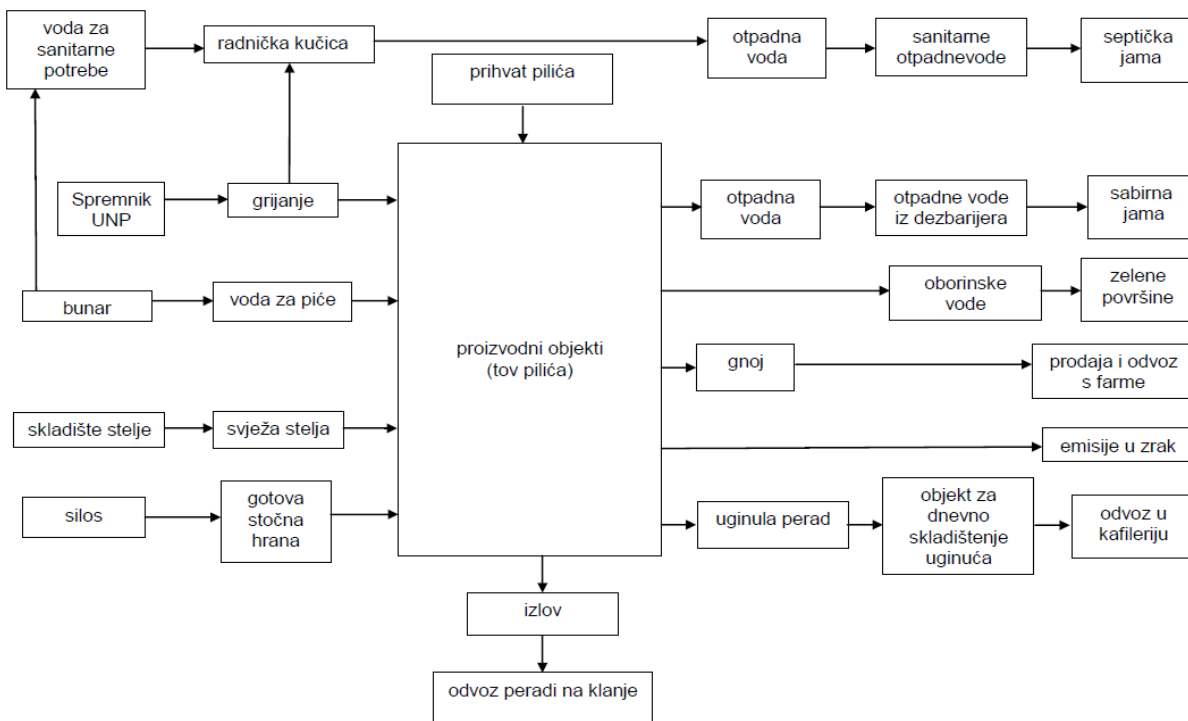
Prilog 3: Pojednostavljena shema procesa na Farmi 13
